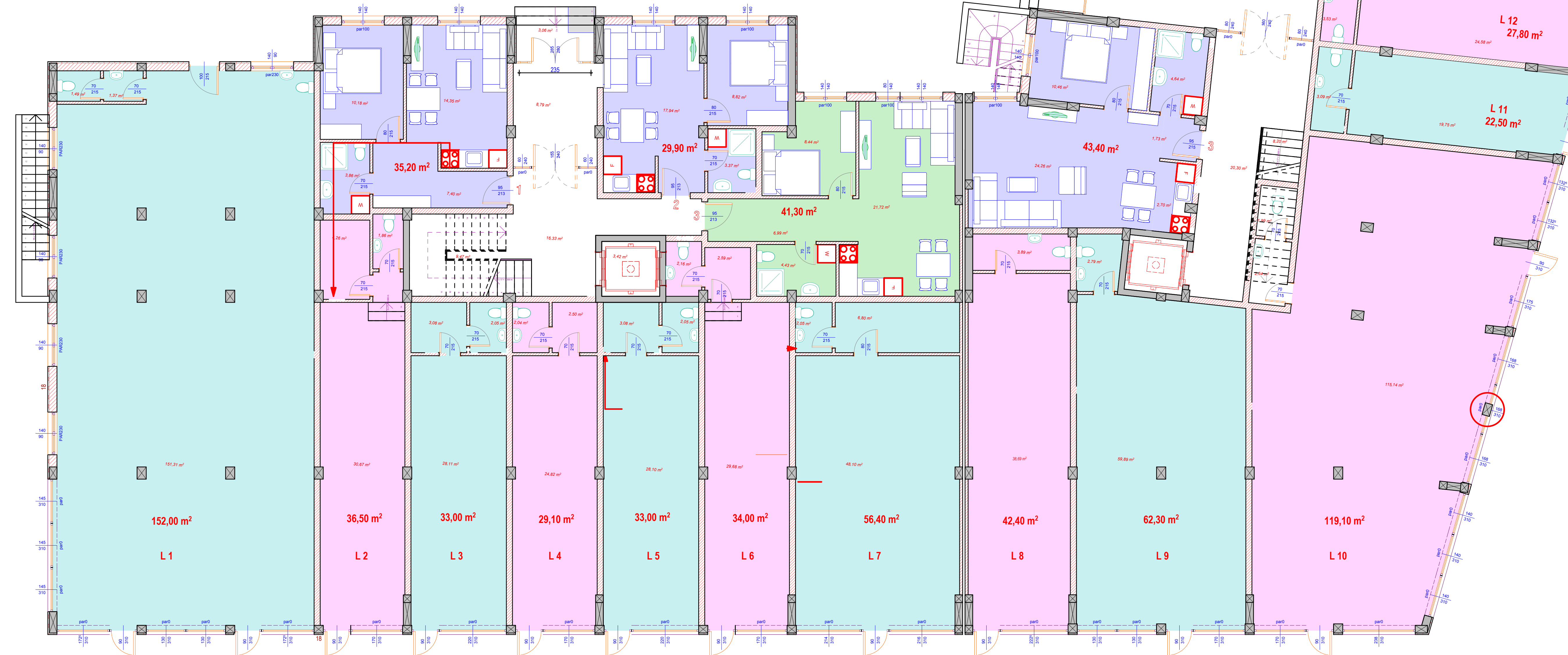
OSNOVA PRIZEMLJA
