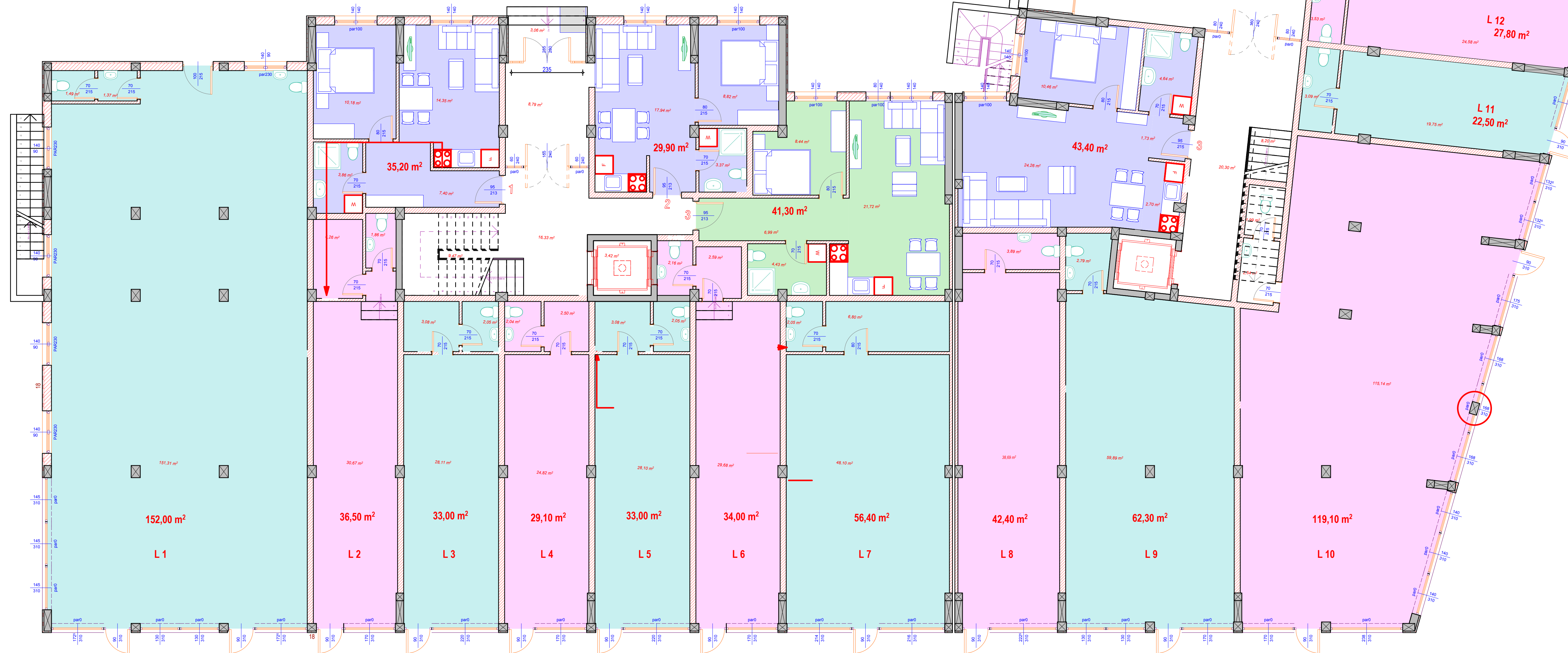
OSNOVA PRIZEMLJA
